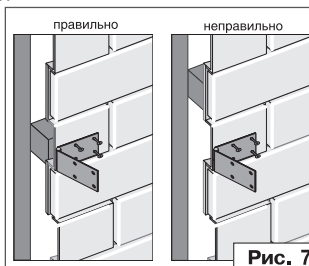
Фасадная панель
