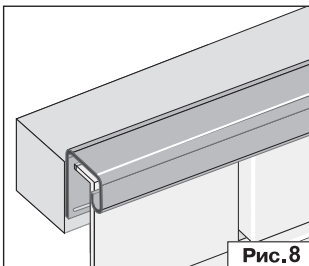
J-профиль
