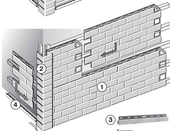
Бордюр
